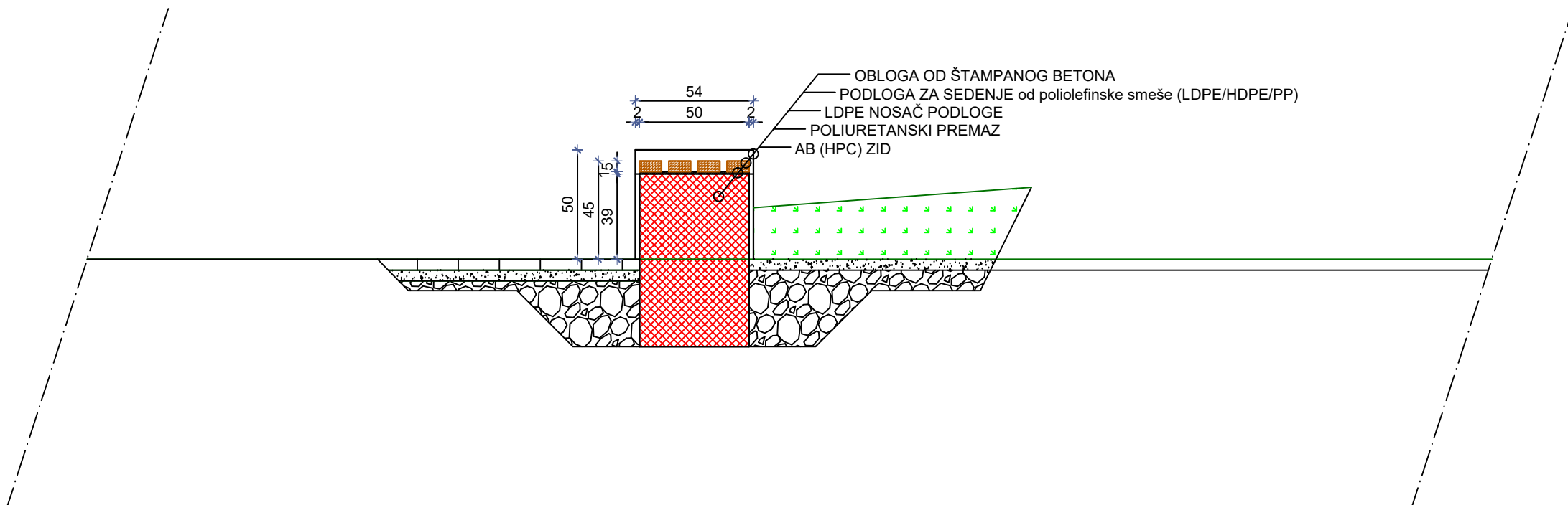
PRESEK ZIDIĆA - ŽARDINJERE SA MESTOM ZA SEDENJE - UPUŠTENA KLUPA
