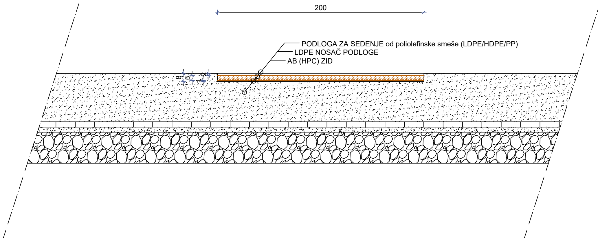
IZGLED ZIDIČA - ŽARDINJERE SA MESTOM ZA SEDENJE - UPUŠTENA KLUPA
