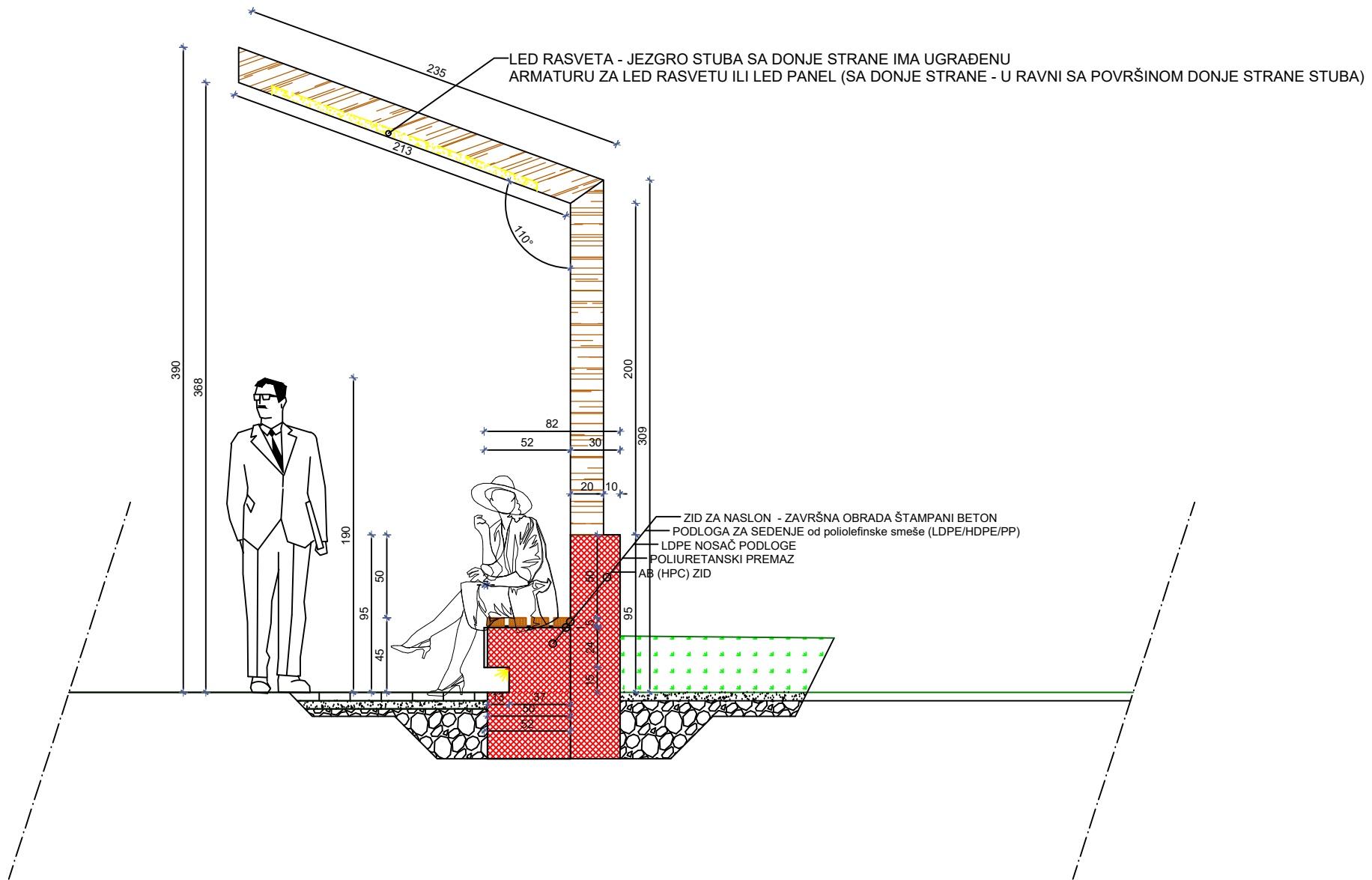
PRESEK ZIDIČA - ŽARDINJERE SA MESTOM ZA SEDENJE I LED RASVETOM NA POZICIJI CENTRALNIH ŽARDINJERA OKO FONTANE
